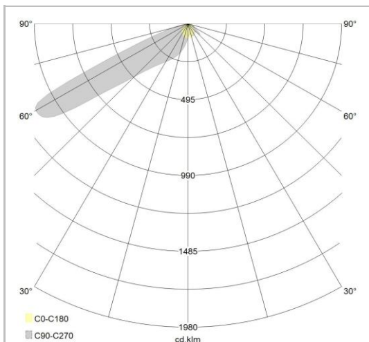
Lumen distributie
