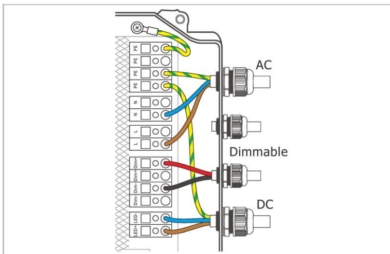
Aansluitschema
