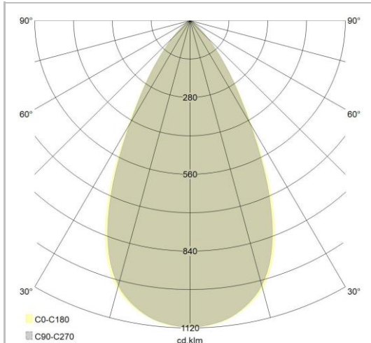
Lumen distributie
