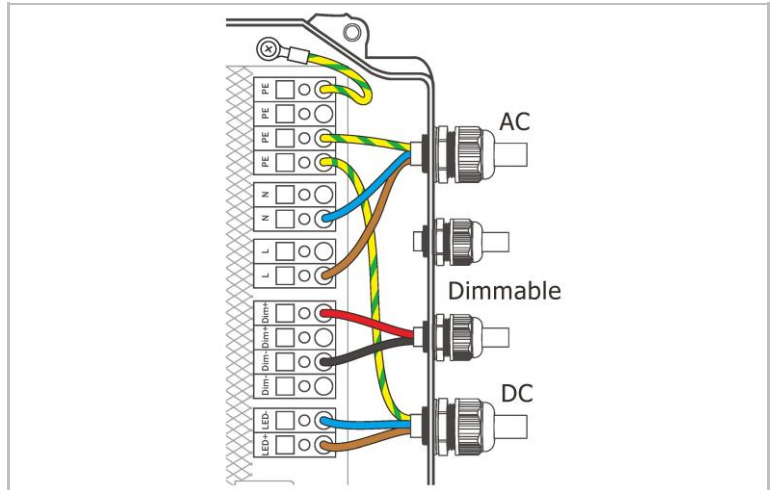
Aansluitschema
